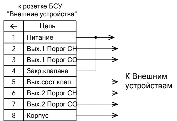
Рисунок Б.4 - Схема распайки вилки подключаемой к разъёму "Внешние устройства" БСУ
