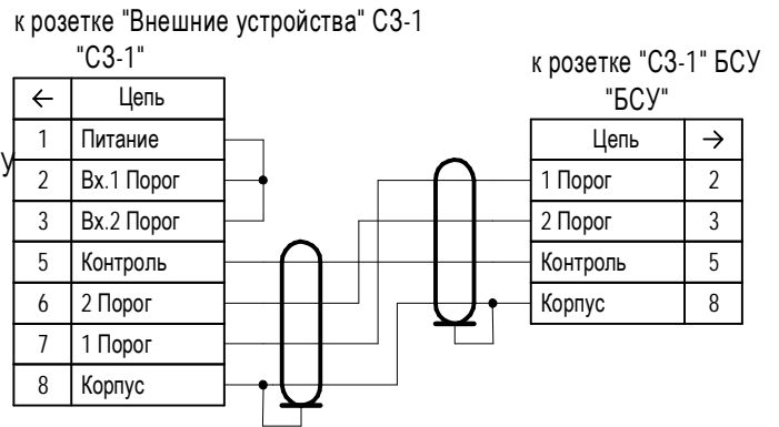
Рисунок Б.2 – Схема кабеля для подключения СЗ-1 к БСУ
