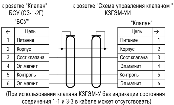
Рисунок Б.3 – Схема кабеля для подключения клапана КЗГЭМ-У
