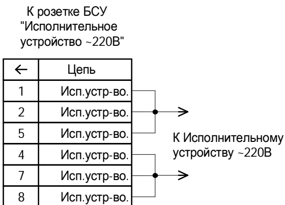
Рисунок Б.5 - Схема распайки вилки подключаемой к разъёму "Исполнительное устройство" БСУ
