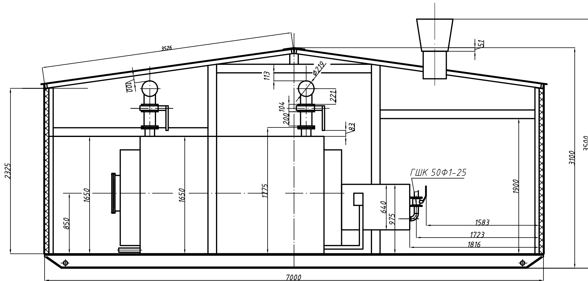
Компоновка котельной ТКМ-4,0 (2,0+2,0)
