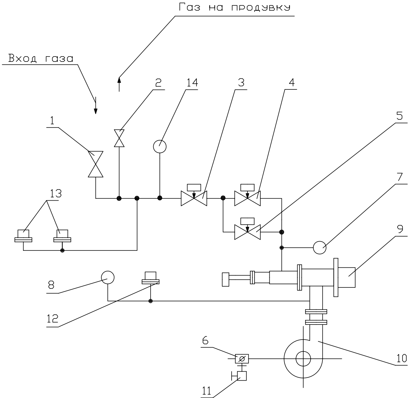
Принципиальная схема газового блока котла КВ-Г-1-115Н (низкое давление)
