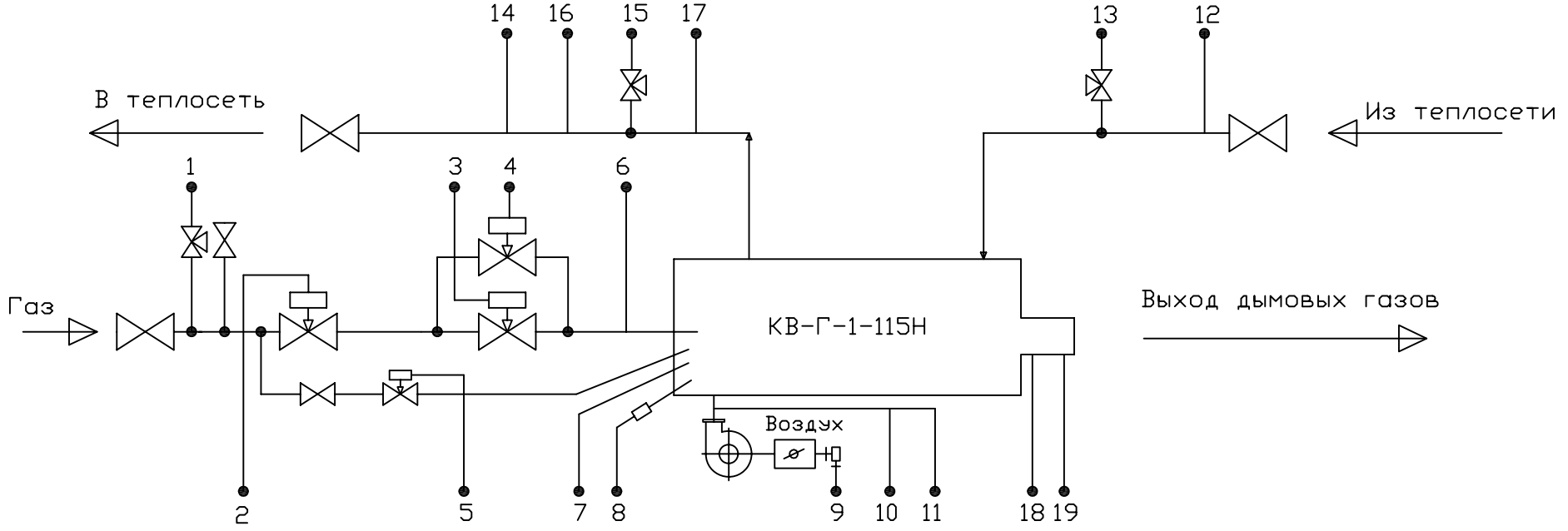
Схема автоматизации котла КВ-Г-1-115Н (среднее давление газа)
