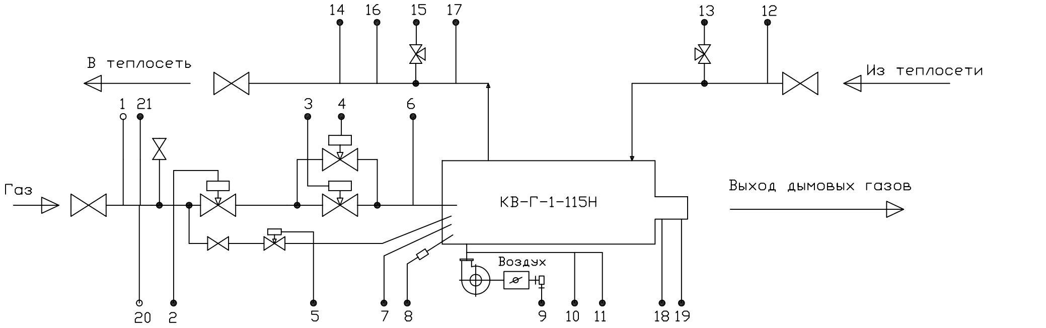
Схема автоматизации котла КВ-Г-1-115Н (низкое давление газа)
