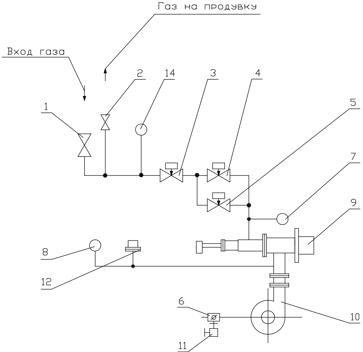
Принципиальная схема газового блока котла КВ-Г-1-115Н (среднее давление)
