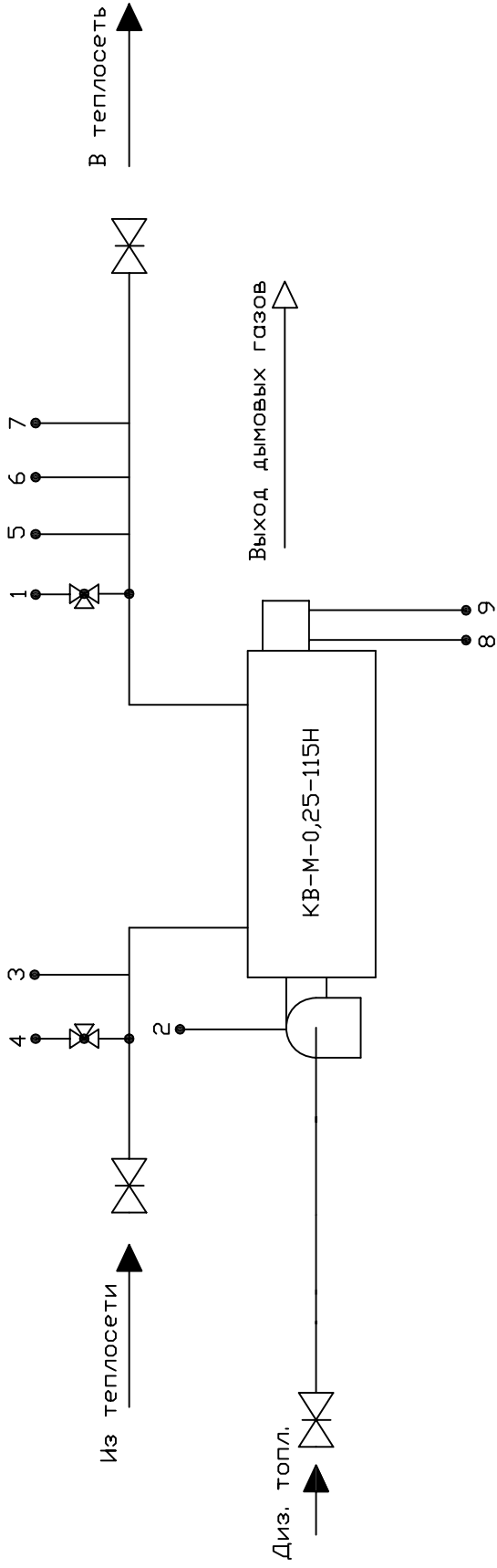
Приложение А Схема автоматизации котла КВ-М-0,25-115Н
