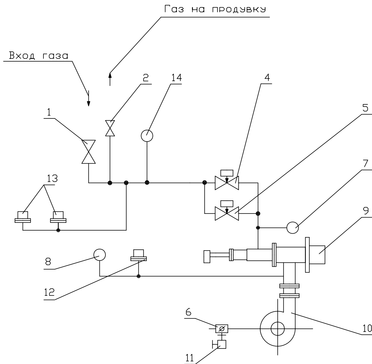
Принципиальная схема газового блока котла KV-G-0,25-115H
